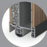
Absenkbare Bodendichtung ohne Schwelle
