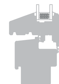
Glasstab profiliert – großer Wetterschenkel
