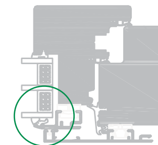
Versatz von Flügel- und Rahmenprofil
