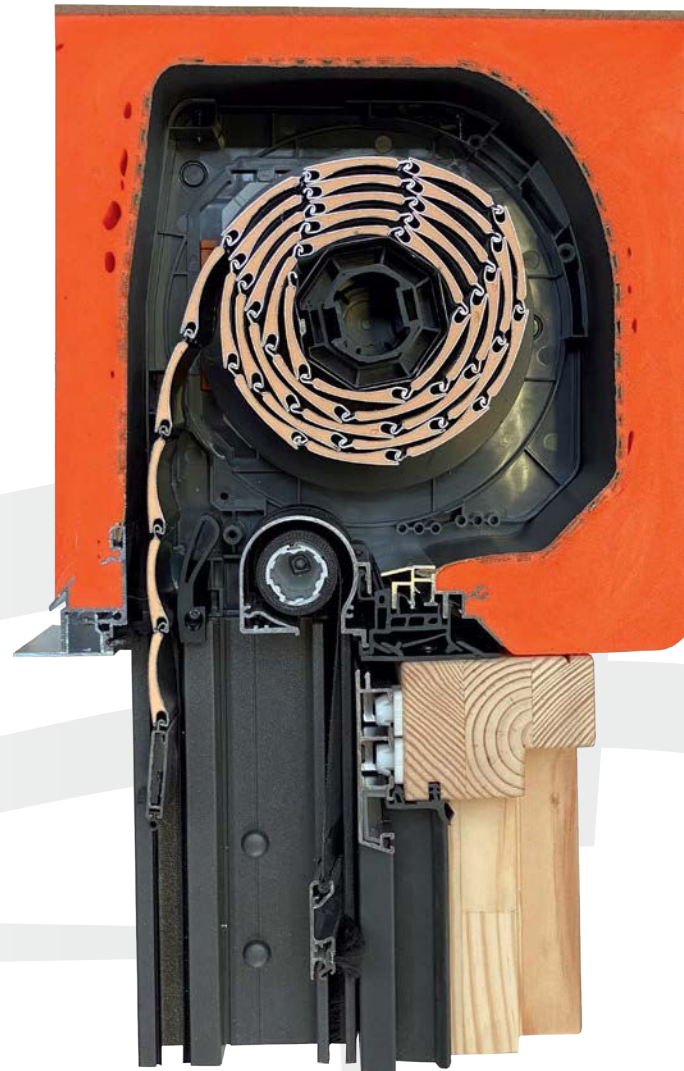
Aufsatzrollladen PURO
