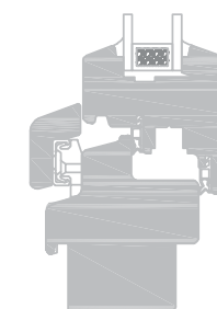
Glasstab gefast – ohne Wetterschenkel
