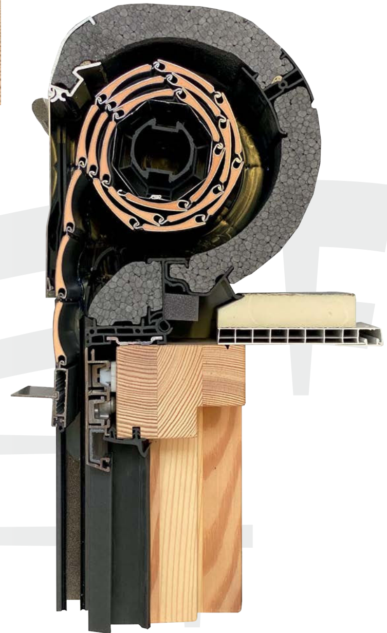
Sanierungsrollladen TERMO
