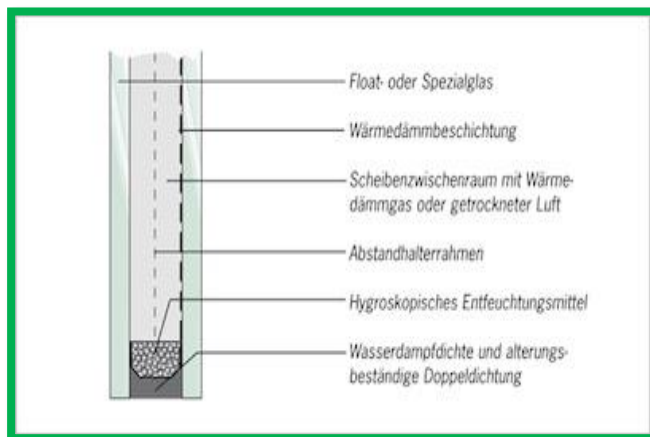
2-fach-Isolierglas
